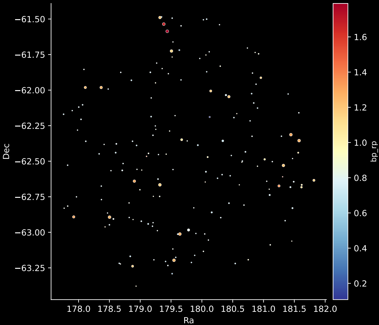
GALAH DR4 Field: [7138] Stars: 171
