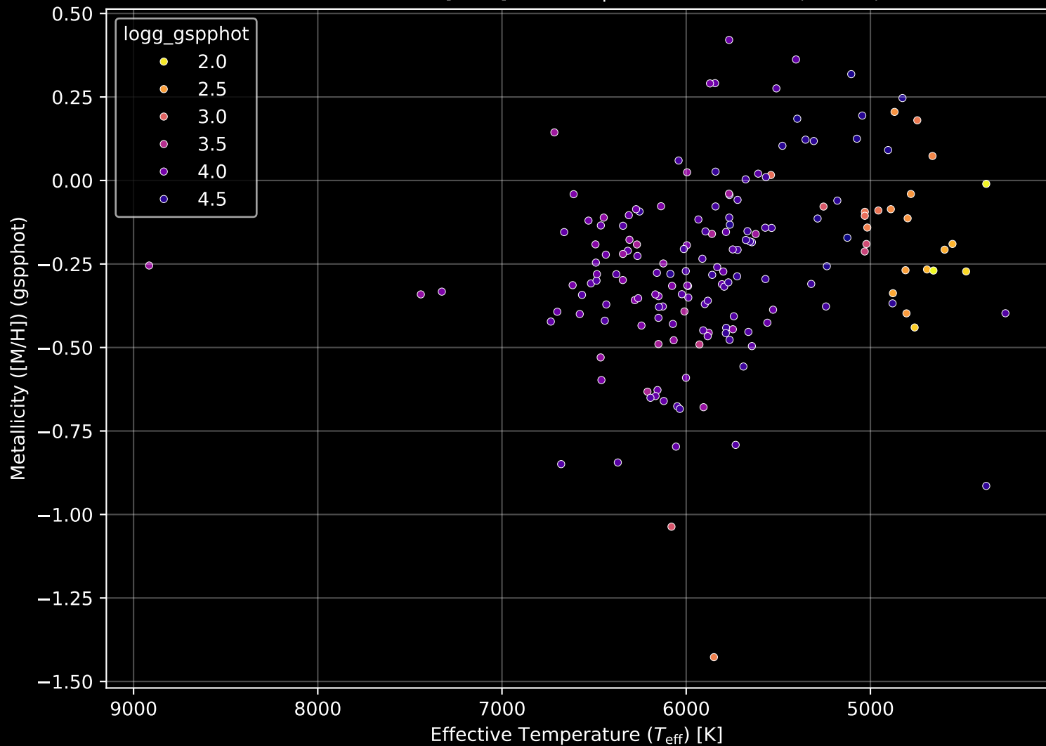
GALAH DR4 Field: [7138] Stellar Population Parameters (n= 171)
