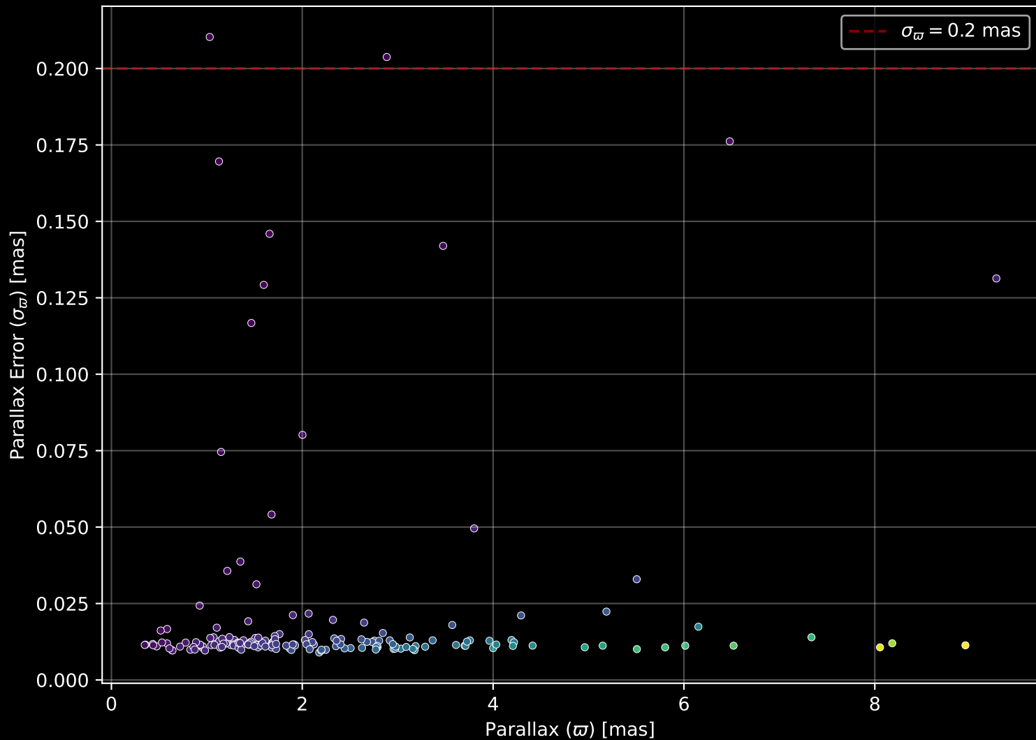
GALAH DR4 Field: [7138] Parallax Quality (n= 171)
