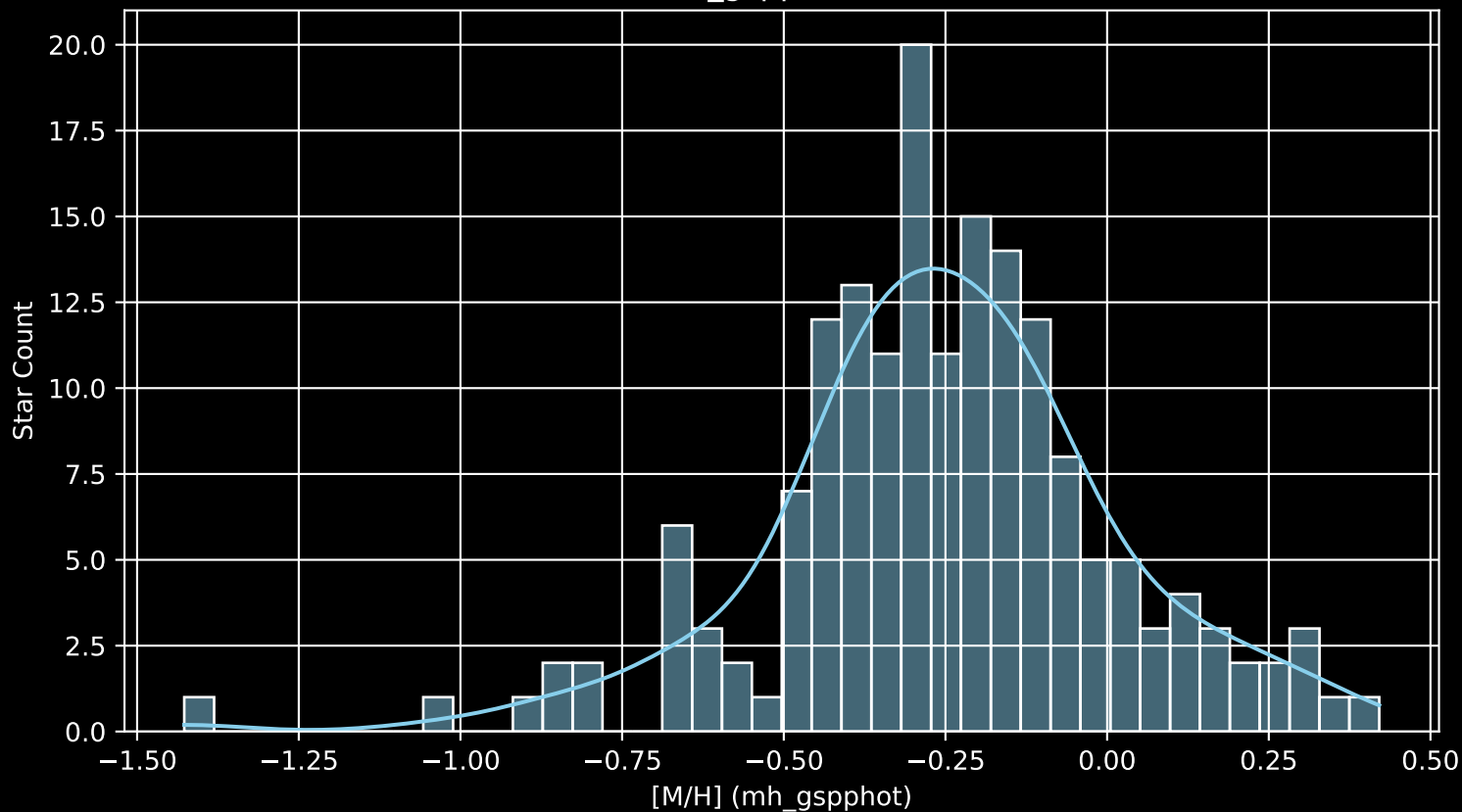
GALAH DR4 Field: [7138] [M/H] (mh_gspphot) (n= 171)
